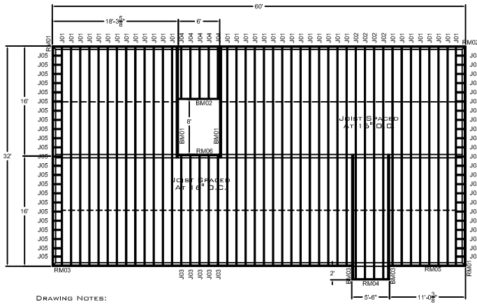
○ JOIST LAYOUT N.T.S.
